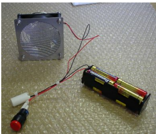
卓上型のファン(AC電源不要)
