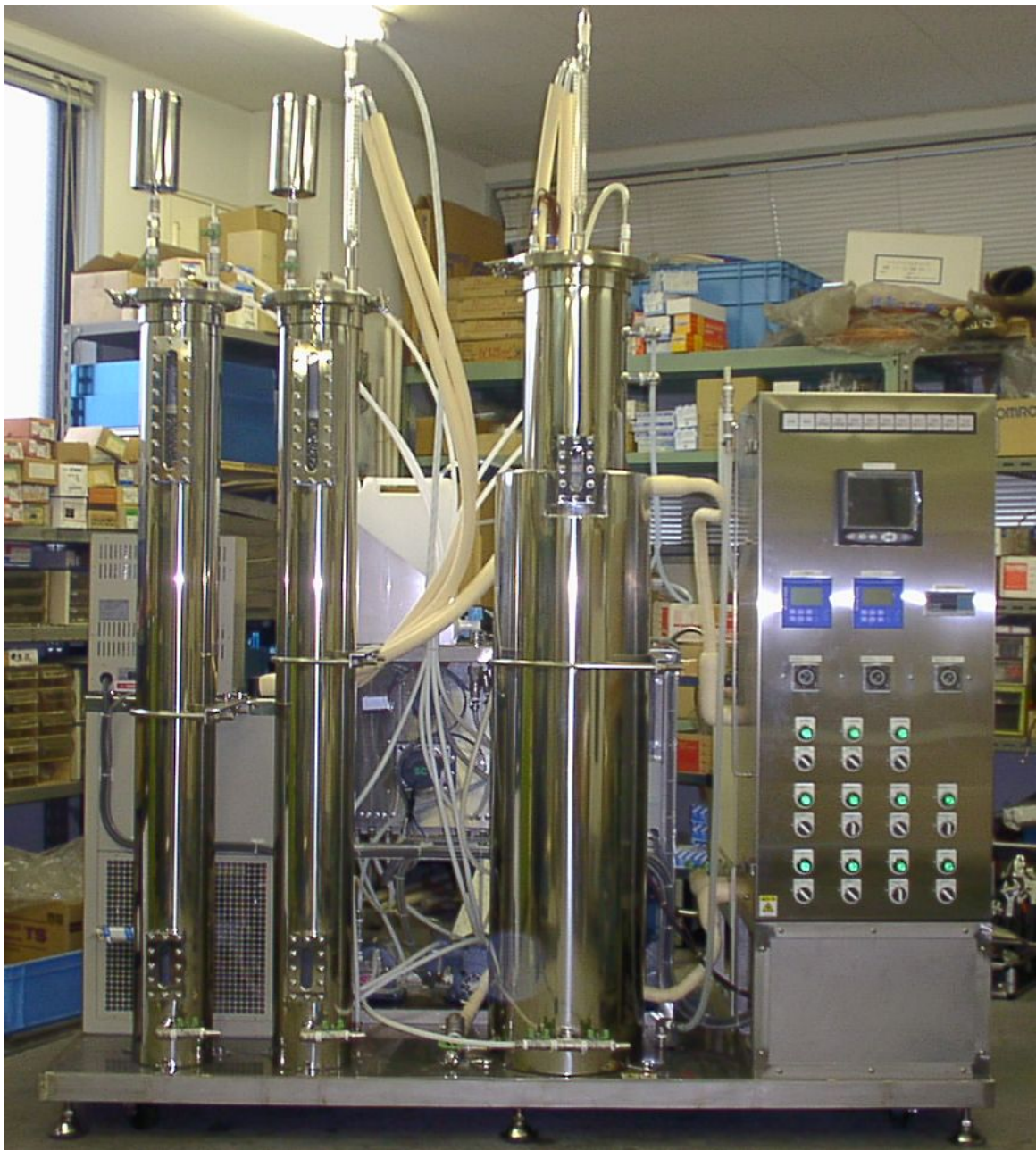
温度・pH・流量等の制御を各反応容器で行う装置(原子燃料サイクル施設)
